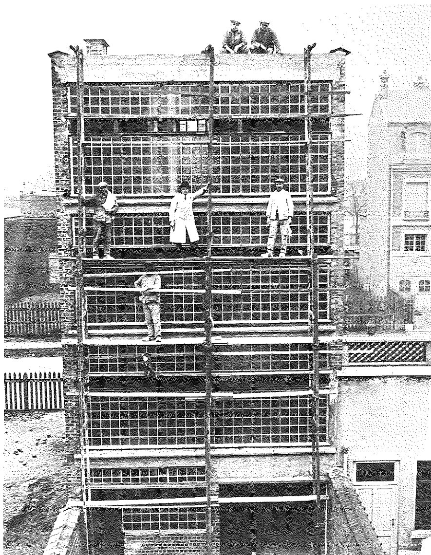
La « Maison de Verre », maison personnelle de l'architecte, rue J.Lejeune à Bruxelles, 1935 : la façade arrière en chantier. Photographie d'époque.
