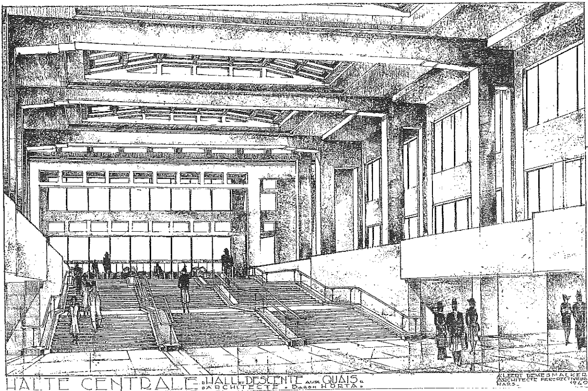
Albert Demesmaeker. Hall et descente aux quais de la Halte Centrale au Cantersteen à Bruxelles (architecte V. Horta), 1940. Fusain sur papier calque, 530 x 740.
