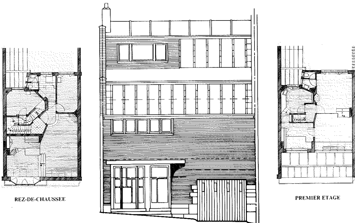
Ateliers d'artistes, rue P.Spaak 4 à Bruxelles, 1930-1931 : plans et élévation de la façade principale. Tirage sur papier. 400 x 800.
