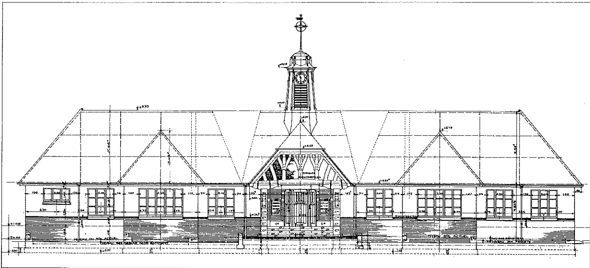
Ferme-école de Waterloo (collaborateur Th. Clément), 1912. Reproductions photographiques des plans d'exécution.
